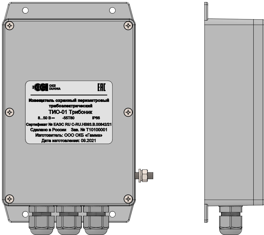
Рисунок 1 – Внешний вид извещателя
