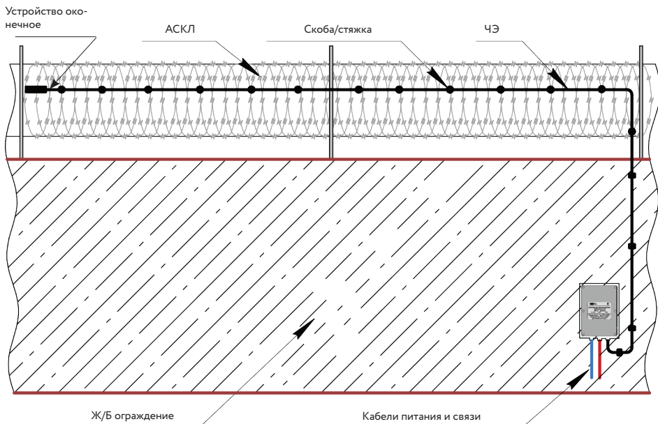
Рисунок А.3 – Конфигурация линии обнаружения вариант 3
