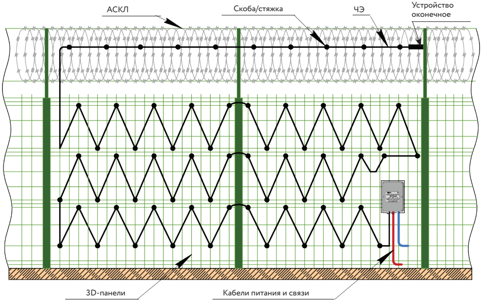
Рисунок А.1 – Конфигурация линии обнаружения вариант 1
