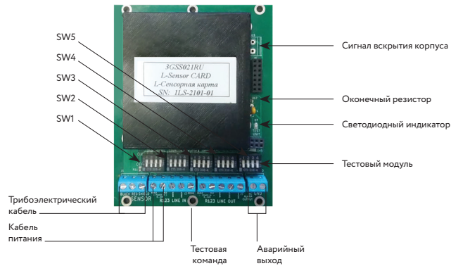
Рисунок 2 – Внешний вид платы БОС
