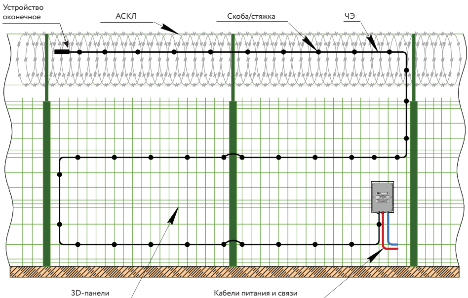
Рисунок А.2 – Конфигурация линии обнаружения вариант 2
